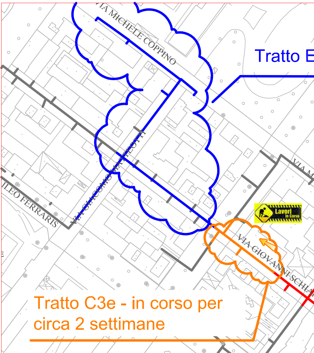
TRATTO DI SCAVO "C3e"
