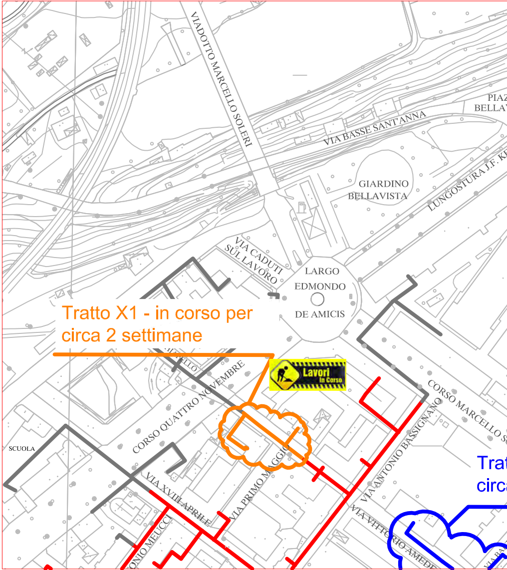
TRATTO DI SCAVO "X1"
