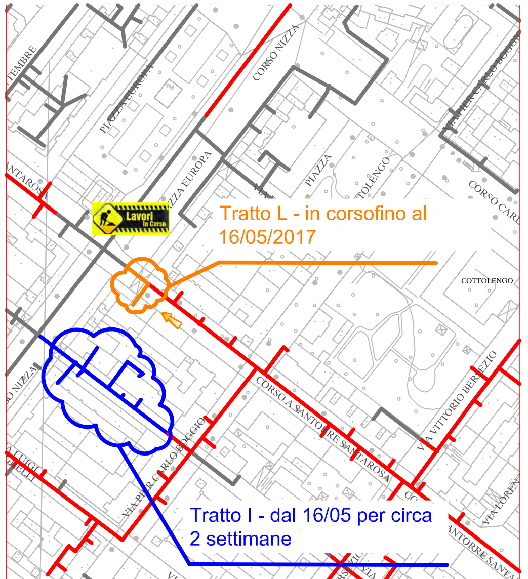
TRATTO DI SCAVO "L"
