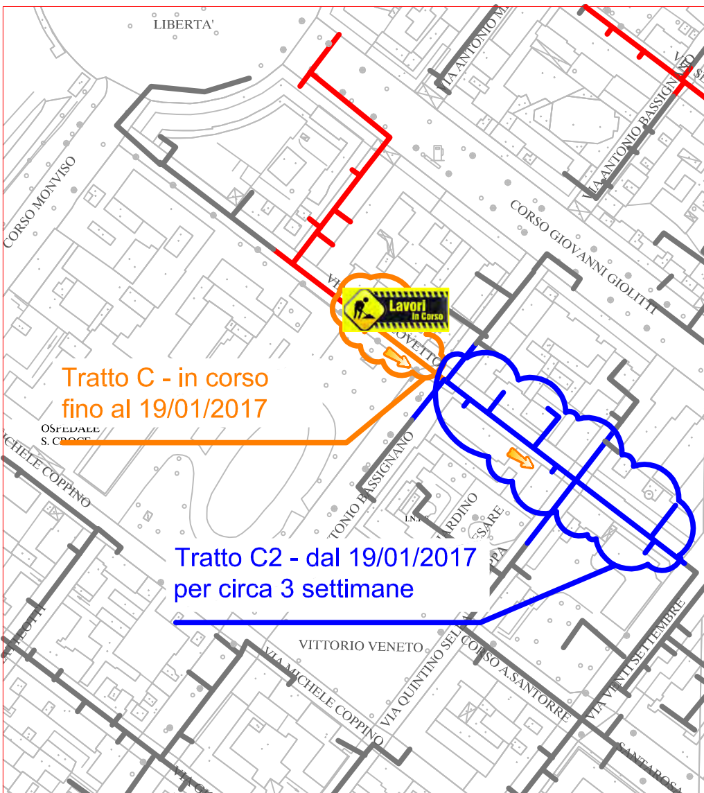
TRATTO DI SCAVO "C"
