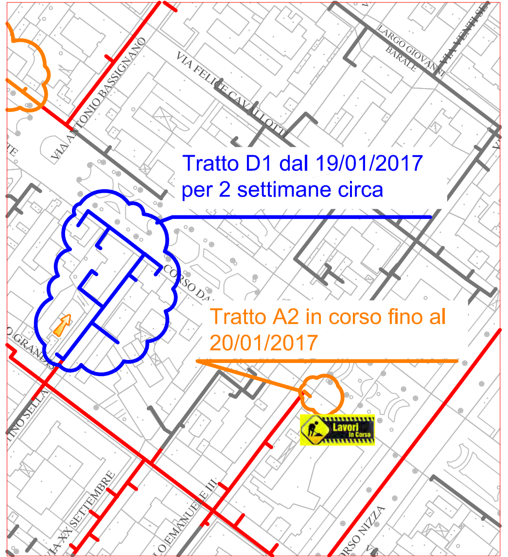
TRATTO DI SCAVO A2"
