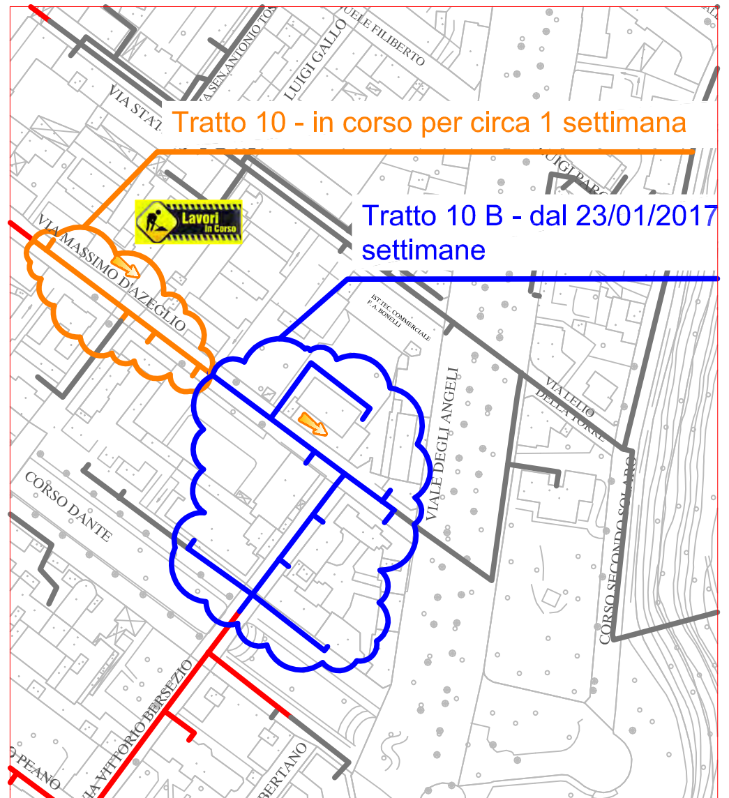
TRATTO DI SCAVO "10"
